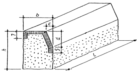
Wymiary krawężnika
